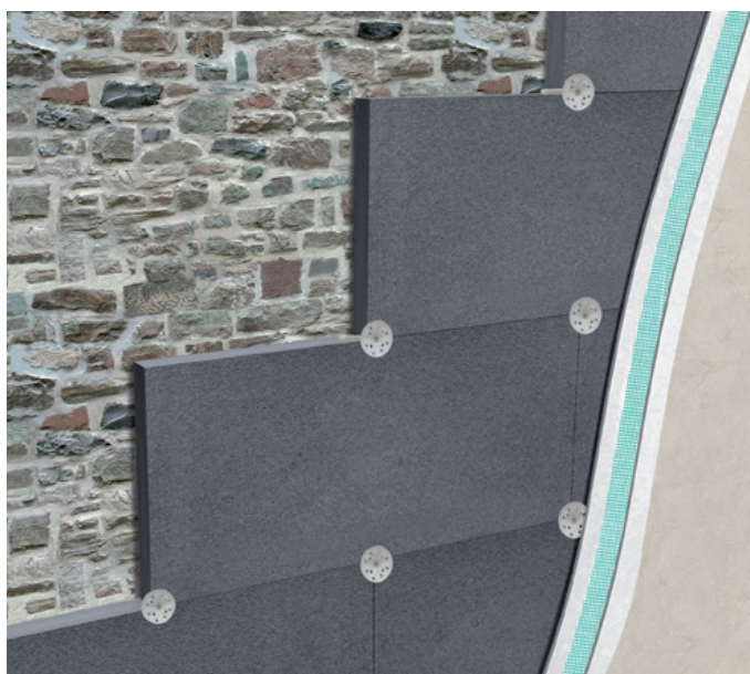
Isolamento a cappotto su parete in pietra
