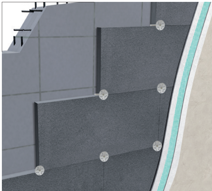
Isolamento a cappotto su parete in calcestruzzo
